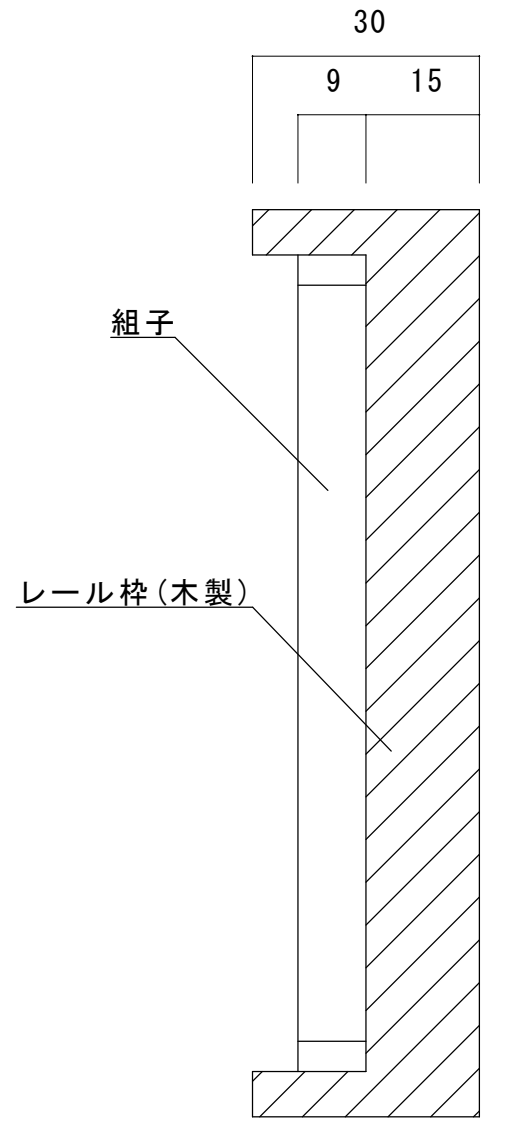
組子断面図 S=1/1
